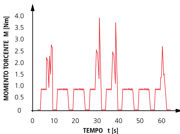
Utensile convenzionale
