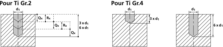
Cycle de rupture de copeaux (par ex. : G73)
