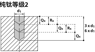
断屑的循环 (例如G73)
